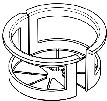
参考斜視図
