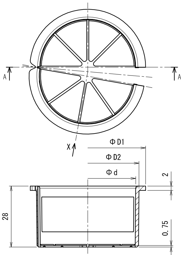
断面 A-A
